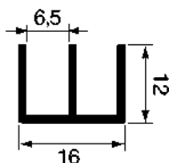
Art. P3556A - Doppia "U"
