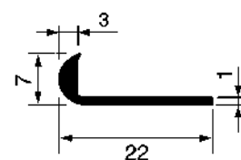
Art. P5503A - Unghietta
