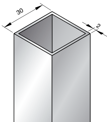
Art. P 0307G-M4 grezzo
