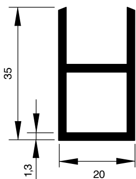
Art. P7301A-M4 argento € 7,70/mt.
