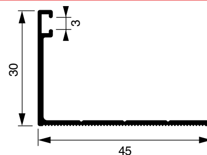
Art. P6020A-B-V - Profilo L
