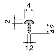
Art. P6001A - Funghetto
