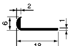
Art. P5502A - Unghietta
