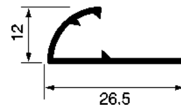
Art. P5097A - Fermapassatoia
