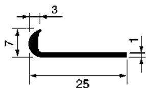
Art. P5504A - Unghietta
