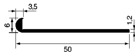
Art. P5512A - Unghietta
