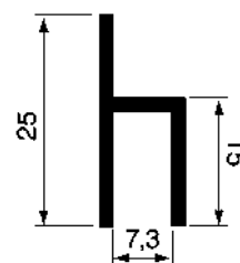
Art. P3532A - Guida Superiore
