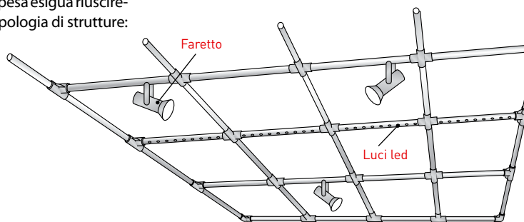
Struttura per controsoffitto aereo e supporto luci con faretti o led
