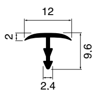
Art. P5520A - Unghietta doppia gobba
