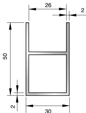
Art. P 2050A-M4 argento
