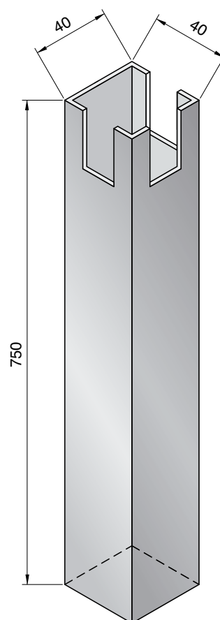
Art. A 43075-00 € 40,95 Gamba in alluminio cm.75 - testa con 3 cave
