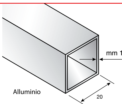
Art. P 4000A-M4 € 6,10/mt. Tubo quadro 20x20mm in alluminio anodizzato satinato argento. Barre da 4 mt
