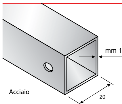
Art. F 4000-0-1 € 7,00/mt. Tubo quadro 20x20 mm in acciaio verniciato color alluminio. Barre da 1,5 mt.
