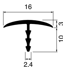
Art. P5521A - Profilo Lato Sagomato
